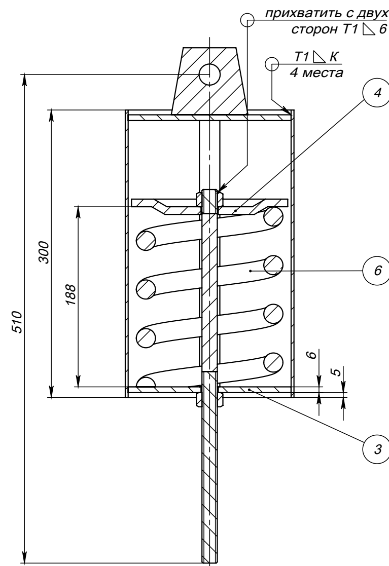
A-A
